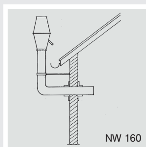
EXA ® -Wandausblas-Set
